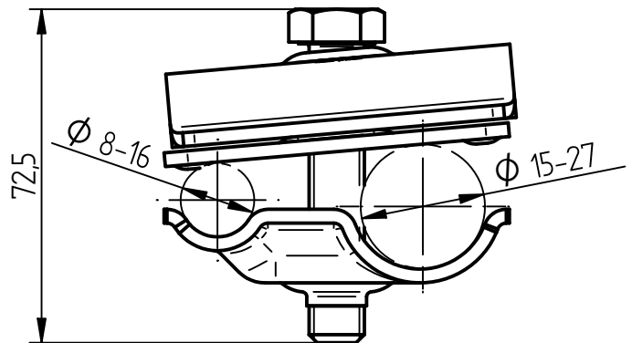
Mögliche Spannbereiche im Unterteil
